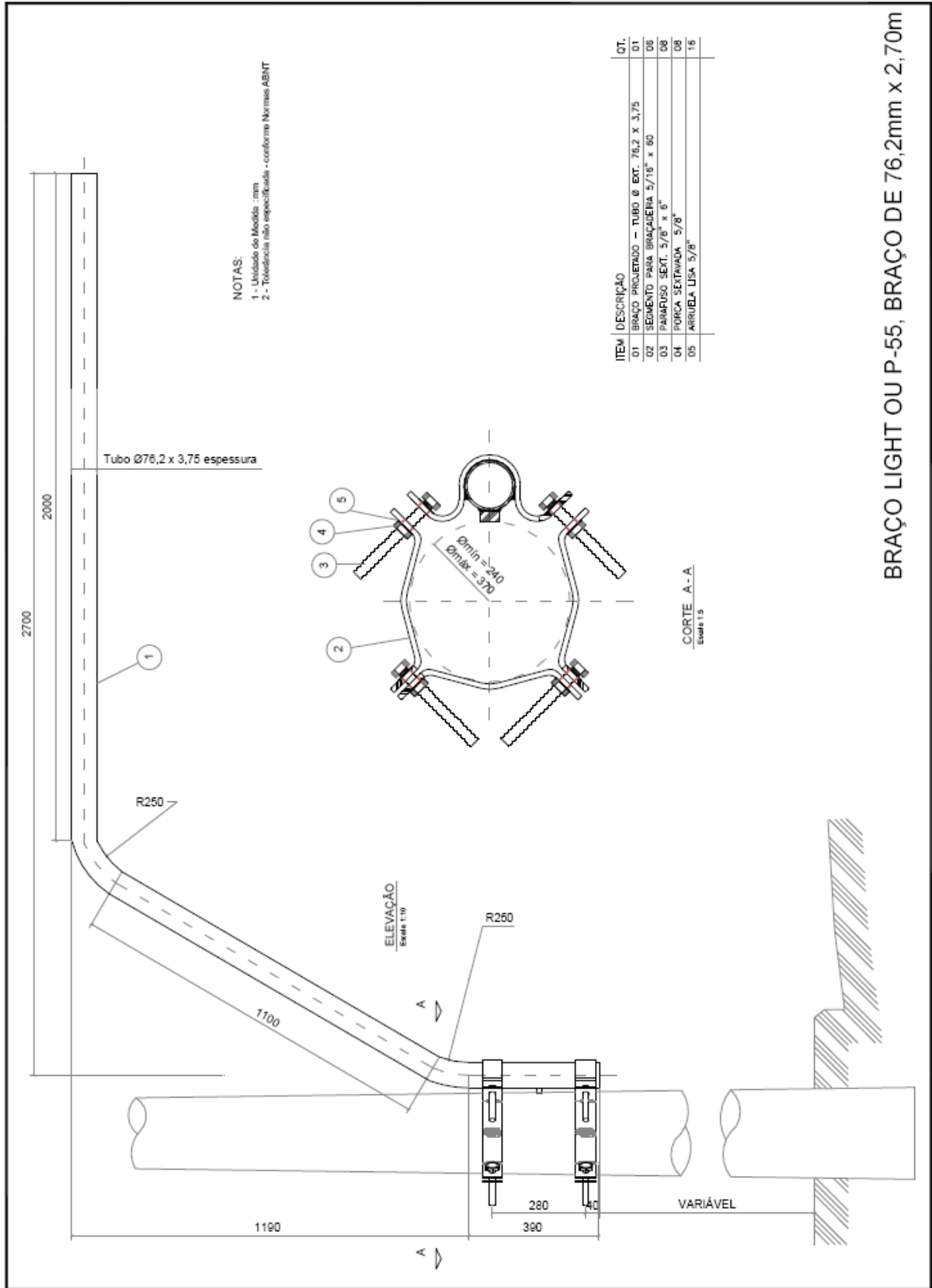
Braço Projetado Light Tipo "P-55"
