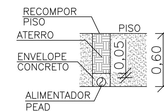
DET. TIPO VALA PARA ALIMENTADOR SEM ESCALA
